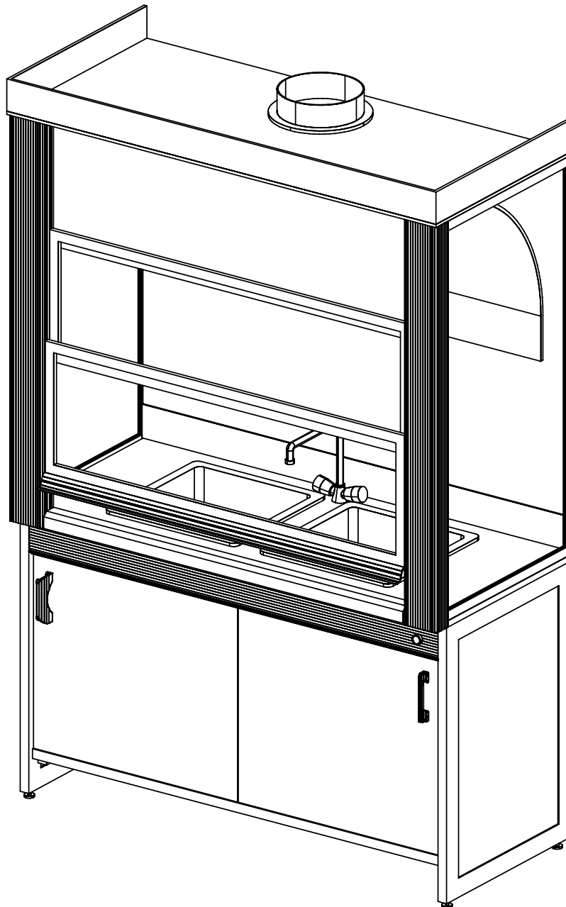
Шкаф вытяжной ЛАБ-PRO ШВ 120.72.225 2V в базовой комплектации
